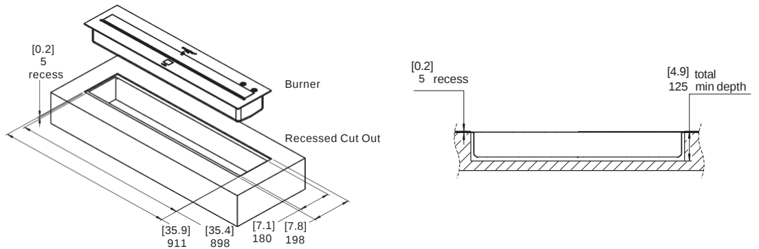
상단 트레이 없이 단채 동일한 높이에서 버너 설치
