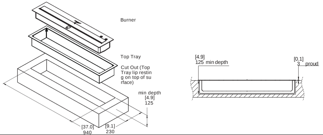
상단 트레이와 함께 버너 설치
